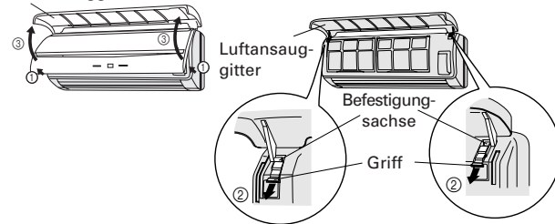
Luftansauggitter
