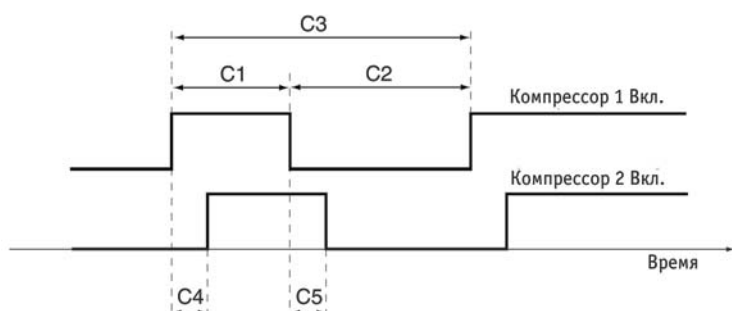
Исполнение с двумя компрессорами
