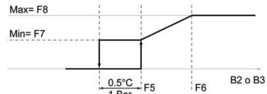
Диаграммы управления вентиляторами внутреннего и наружного блоков
